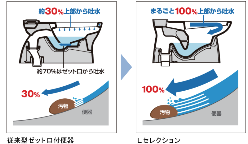
従来型ゼット口付便器
